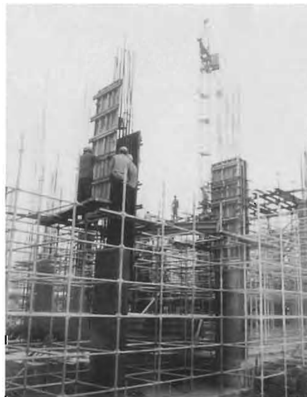
Hệ thống giáo Hàn Quốc tại công trình Tháp Hà Nội South Korea scaffolds system at Hanoi Towers
