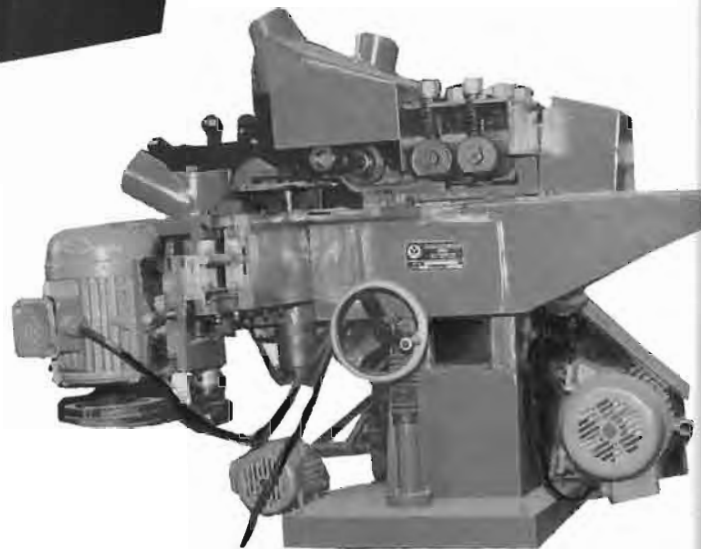
Máy bào 3 mặt Three side planer
