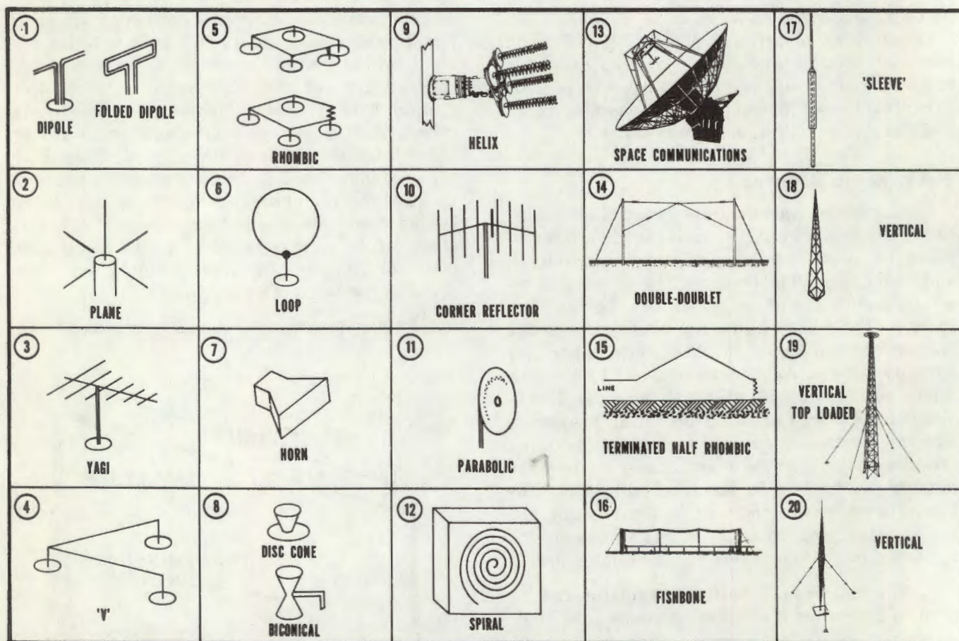
Figure 6-3. Radio antennas.
