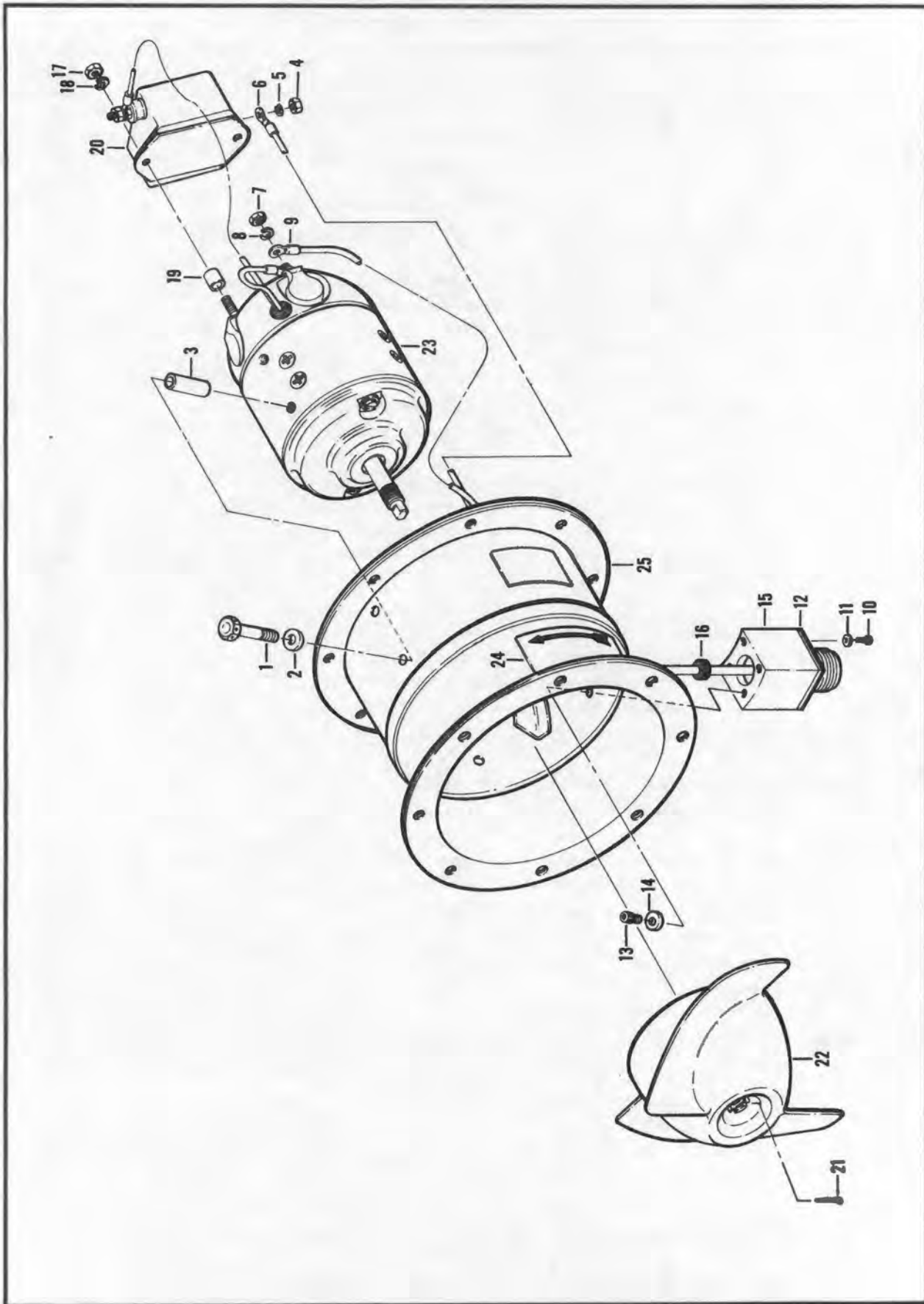
Figure 268E. Fan Vaneaxial, 27 Volt Dc
